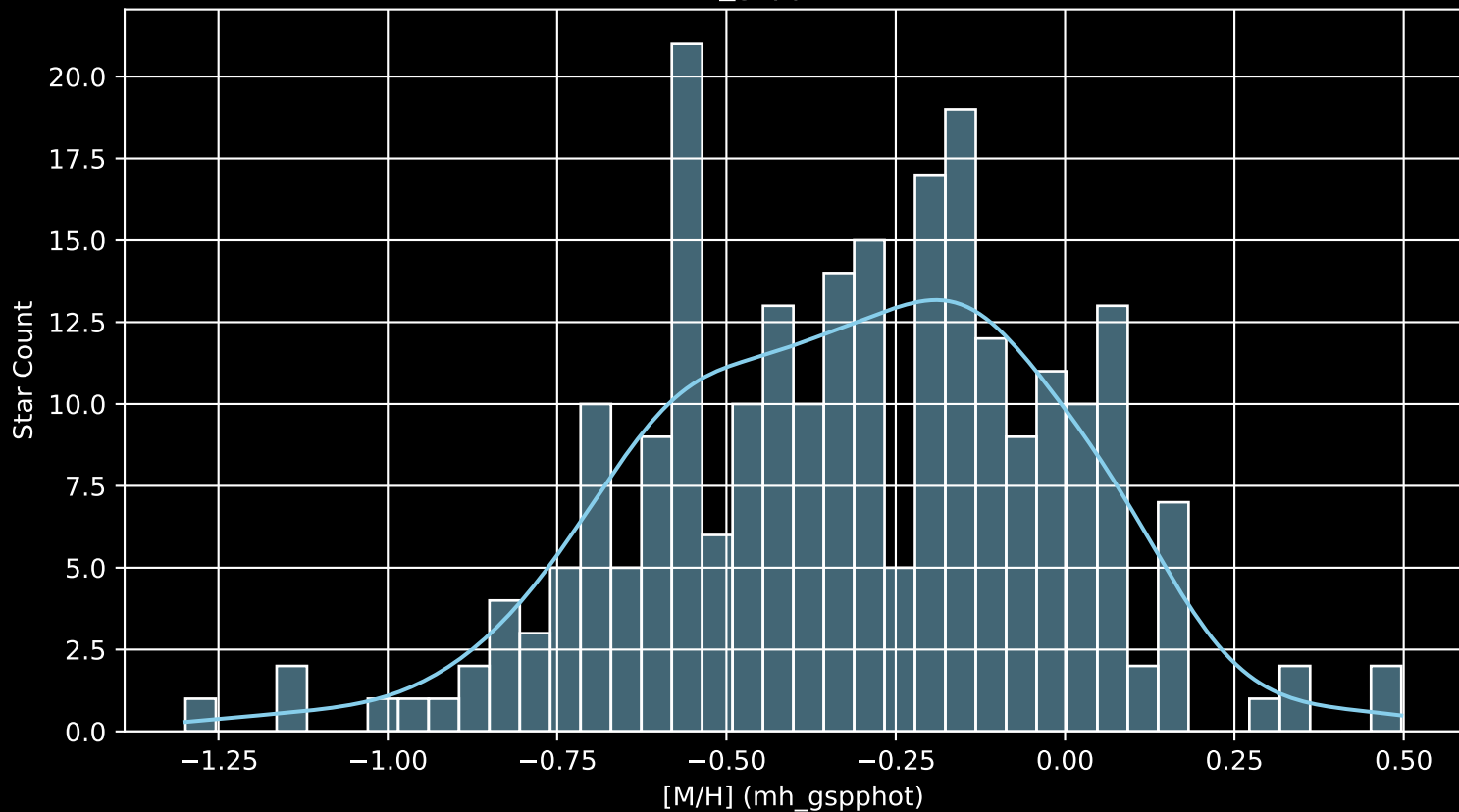
GALAH DR4 Field: [7169] [M/H] (mh_gspphot) (n= 243)
