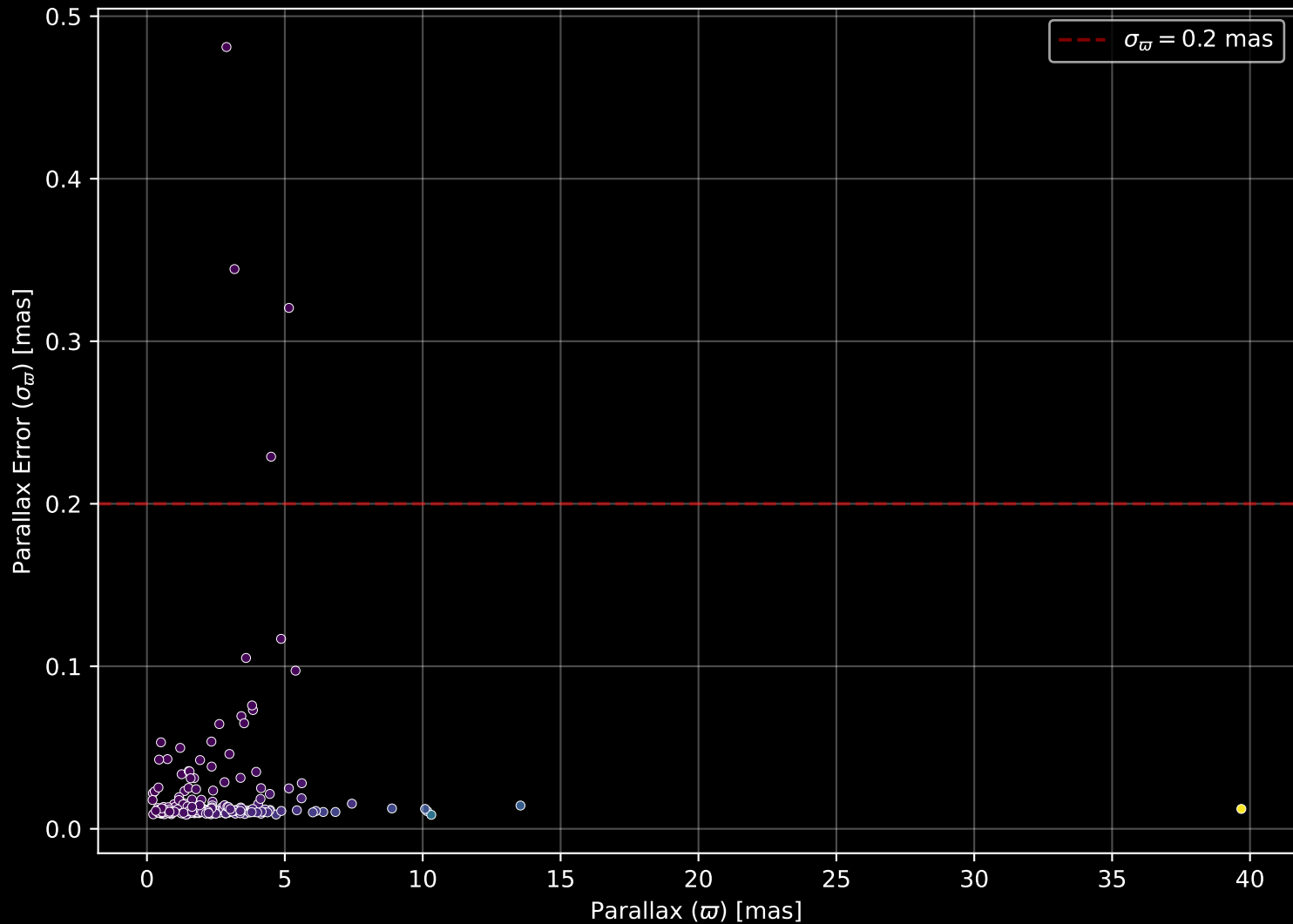
GALAH DR4 Field: [7169] Parallax Quality (n= 246)
