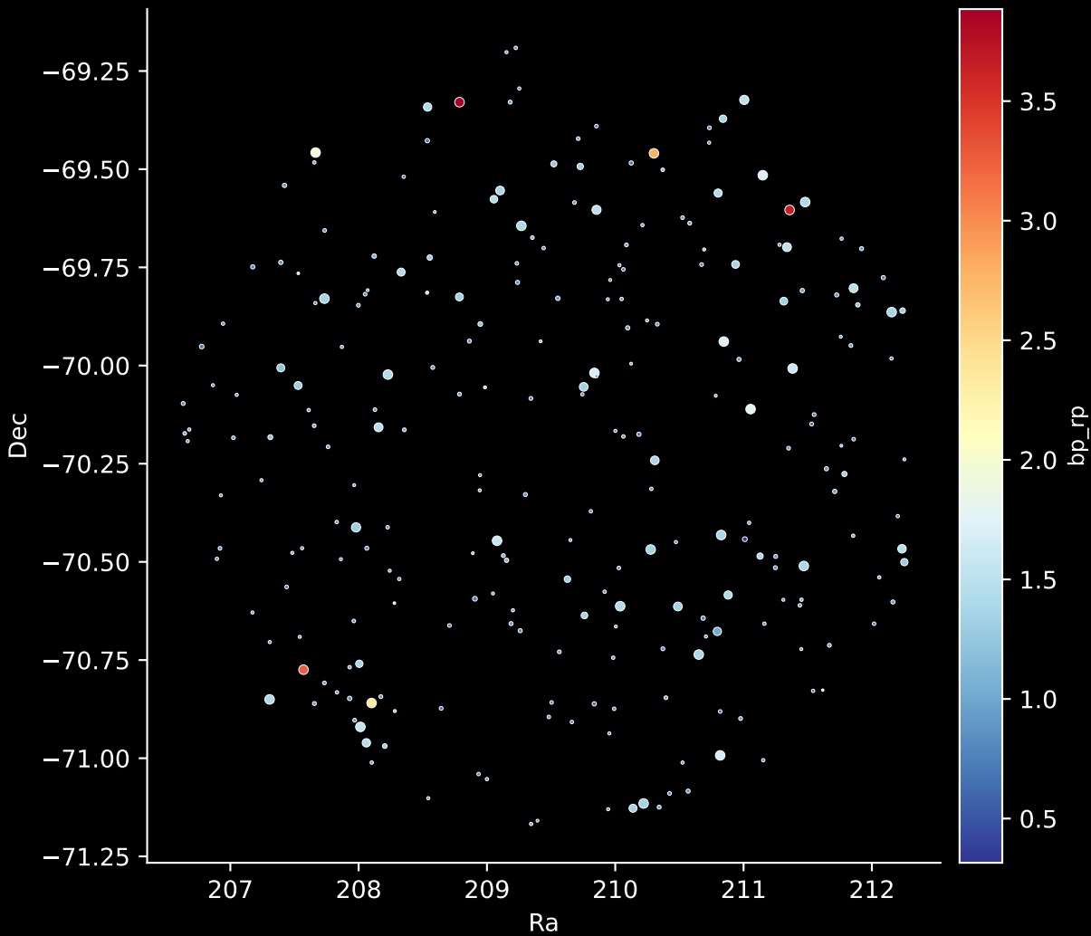
GALAH DR4 Field: [7169] Stars: 246
